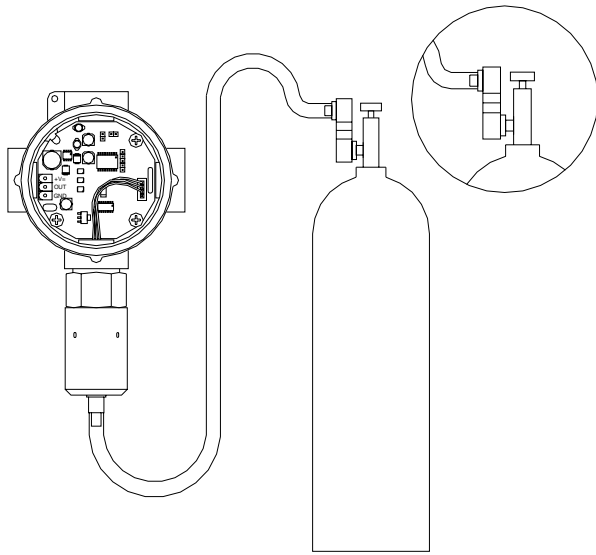
Fig. 3: Cómo aplicar el gas de prueba para el transmisor.
